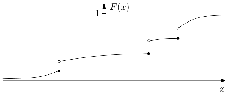
Abb. 2.1: Eine Verteilungsfunktion.
