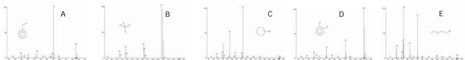
Massenspektren
